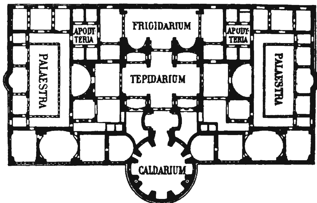
Fig. 6. — Plano de las termas de Caracalla.
